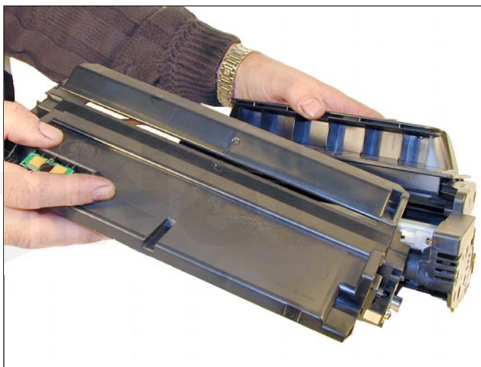
35. Instale la sección de desperdicio en la cubierta lateral fija que está en la cavidad de suministro. Este es un proceso difícil las primeras veces, pero después es mucho más sencillo. La mejor manera de realizarlo es halar con mucho cuidado la cubierta lateral hacia afuera, y deslizar la sección de desperdicio hacia arriba y hacia adentro, hasta que todo este alineado. Las primeras veces, es mucho más fácil decirlo que hacerlo. Pero lo dominará.
