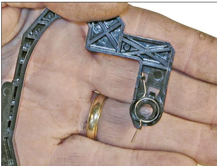
40. Instale el resorte en el brazo de la cubierta del cilindro. Hale la cola superior del resorte hasta que esté en la muesca del eje del brazo.
