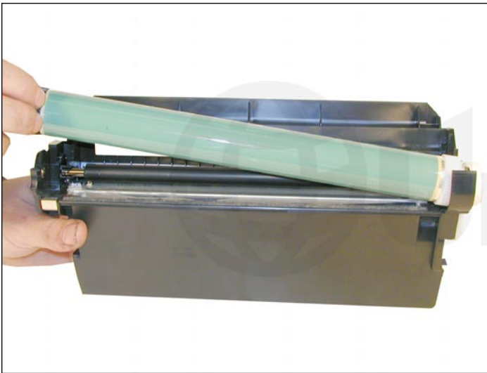
10. Remueva el cilindro.
