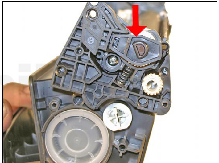
33. Instale la cubierta angular del MRS. Asegúrese que el agujero angular en la cubierta este igual que el lado angular del imán en el ensamblaje del MRS.
