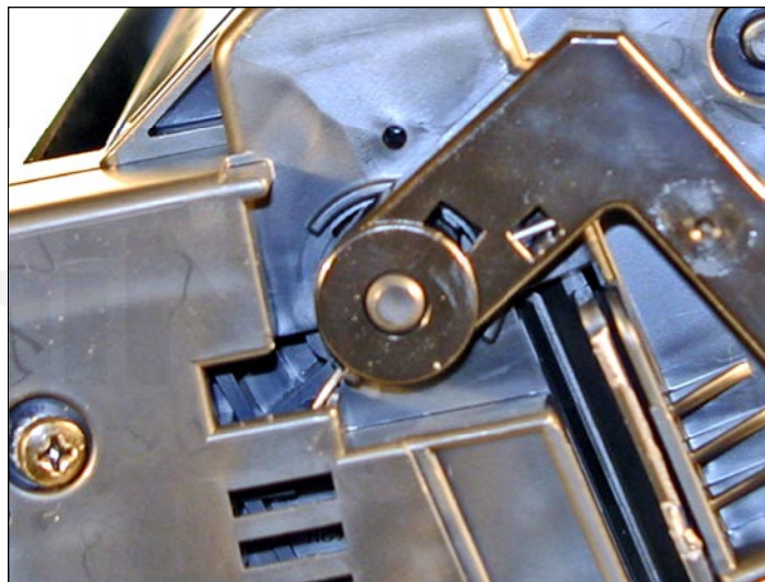
41. Instale el brazo en el cartucho. Libere el resorte de la muesca de manera que la cola embone como se muestra.
