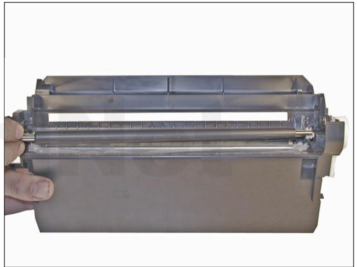
11. Remueva el PCR.
