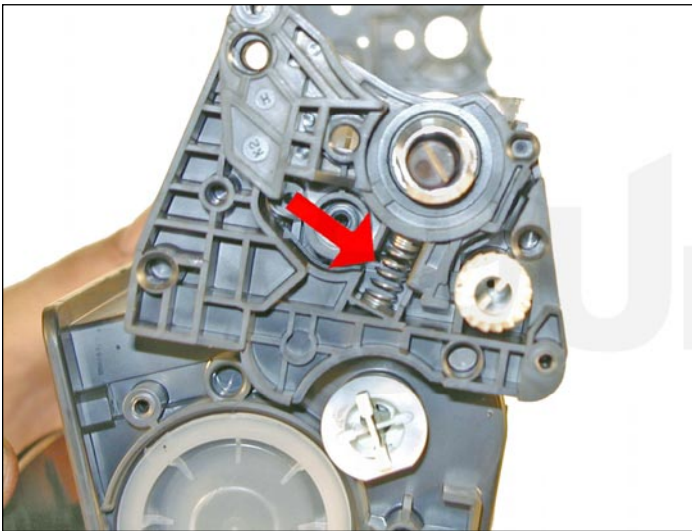
30. Instale el soporte y el resorte.
