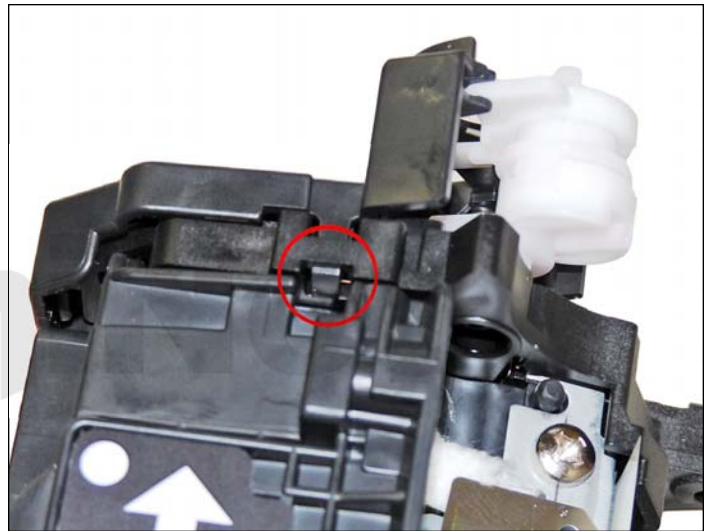
26. En el lado opuesto de la cubierta lateral remueva el único tornillo que hay y presione la lengüeta para liberarla.
