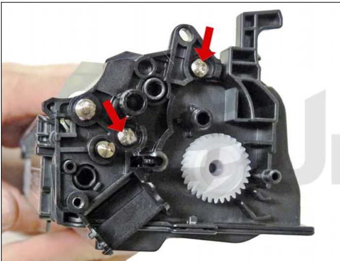
24. Remueva los dos tornillos internos y el engranaje de la cubierta lateral interna.
