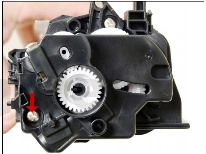
46. Instale la cubierta del engranaje de la cubierta lateral y atornille.
