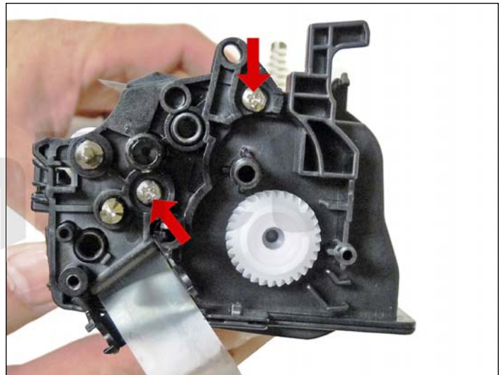
44. Instale el engranaje interior de la cubierta lateral y los dos tornillos.
