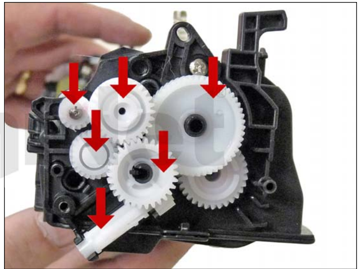
23. Remueva todos los engranajes como se muestra a excepción del engranaje de cuchilla mezcladora. Este está junto con la cuchilla mezcladora, y es muy difícil colocarlo de nuevo adecuadamente.
