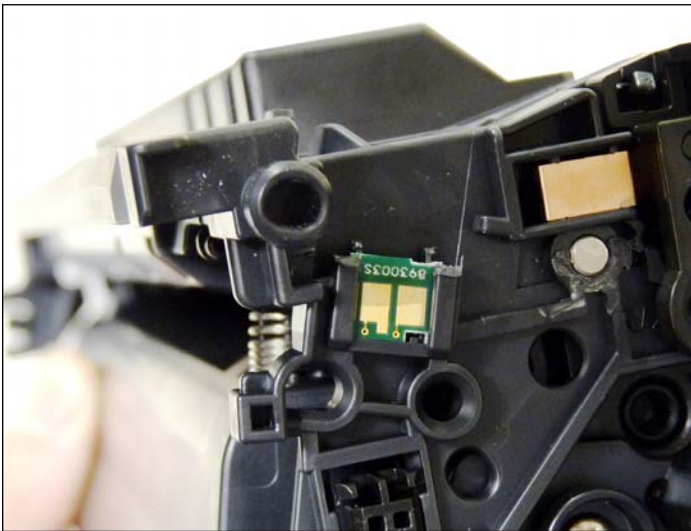
52. Remueva y reemplace el chip. Si el chip nuevo queda suelto en la ranura, cierra los bordes superiores con un poco de pegamento caliente.
