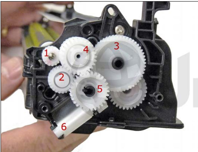
45. Instale los engranajes en el orden mostrado. Si instala un sello, deslice el sello através del engranaje de toma y envuelva la parte floja en el rodillo.
