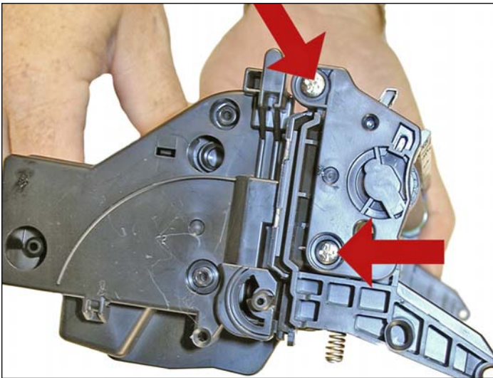
17. En el lado de contacto, remueva los dos tornillos y la cubierta lateral.
