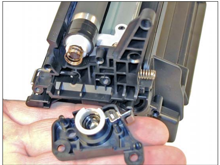
17. En el lado de contacto, remueva los dos tornillos y la cubierta lateral.
