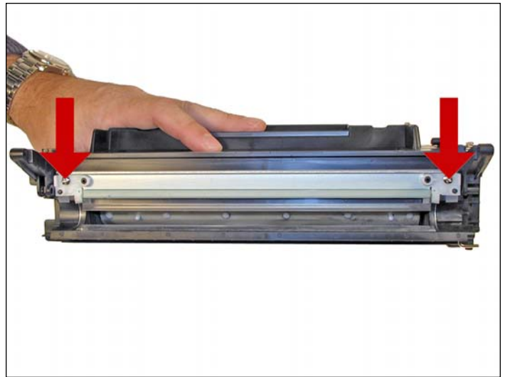
19. Remueva los dos tornillos y la cuchilla dosificadora.
