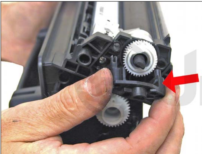
19. En la tolva de tóner, hacer palanca para levantar y sacar la tapa del rodillo magnético.
