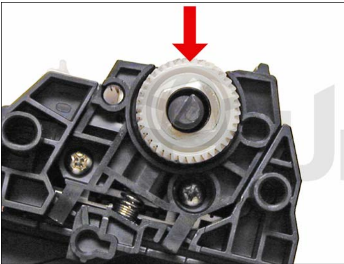
34. Montar el engranaje de impulsión del Rodillo Magnético.
