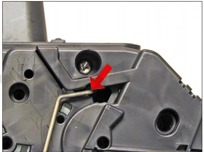
41. Montar la barra metálica de la tapa del OPC en ambos lados del cartucho.
