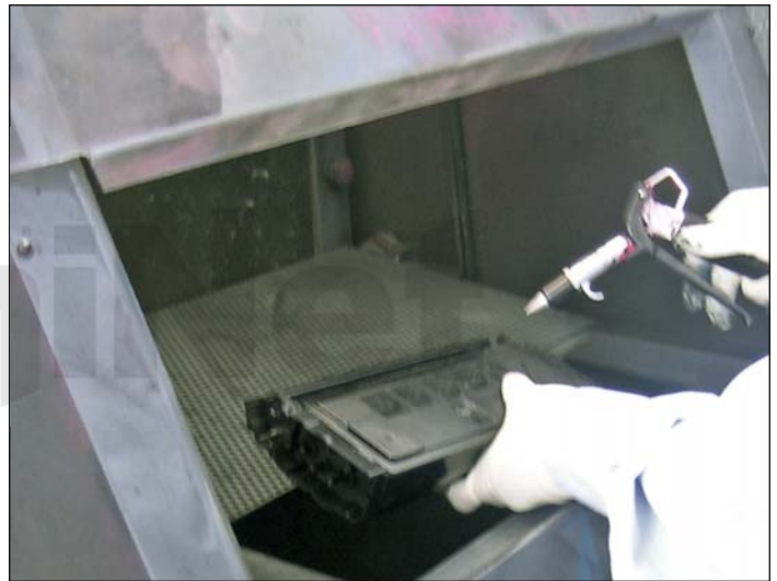
20. Limpe todo o cartucho utilizando ar comprimido ou aspirador de toner. Insira 255 gramas de toner para uso em Xerox WorkCentre 4118 e monte novamente o cartucho seguindo os passos aqui descritos na ordem reversa. Antes de reinstalar a tampa lateral do lado das engrenagens, encaixe o novo Smartchip e verifique se está bem fixo no local.
