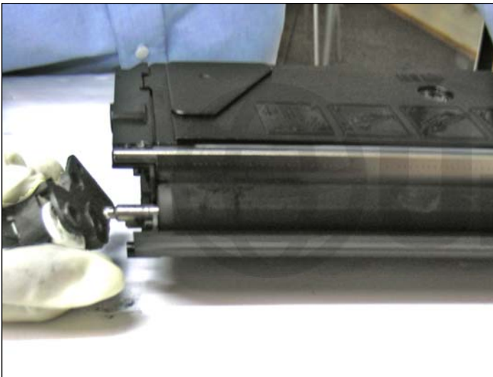
7. O suporte do rolo revelador já removido.
