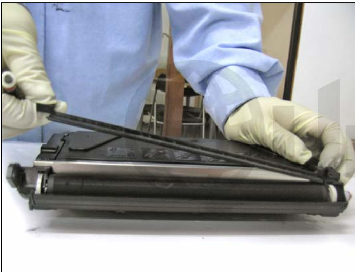
5. Levante e remova a lâmina dosadora.
