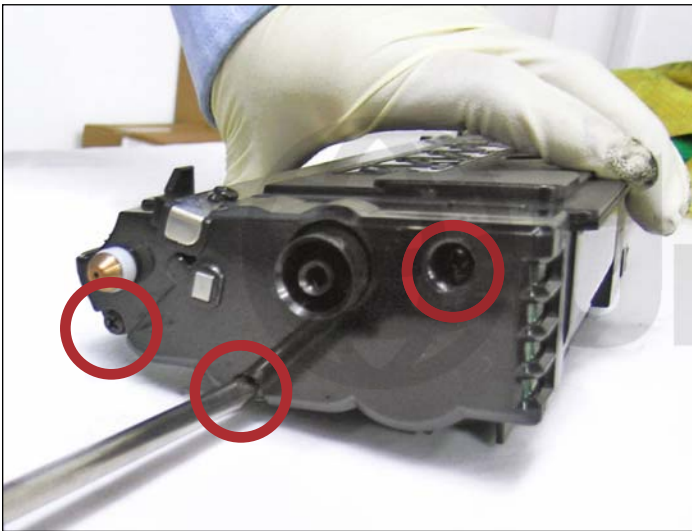
9. Remova os três parafusos do lado das engrenagens, como mostrado.
