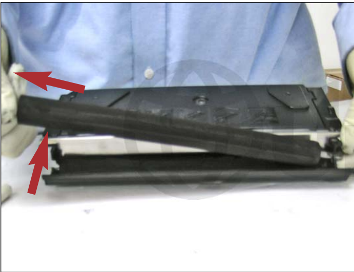
17. Levante e retire o rolo revelador da forma apresentada na foto.
