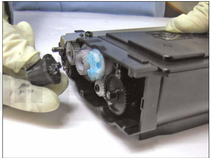
12. Remova a engrenagem preta externa, como mostrado.
