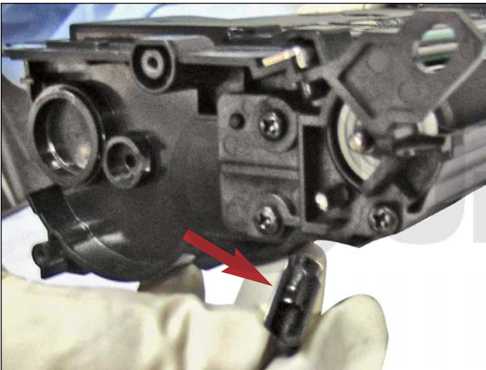
3. Retirar el engranaje de extensión próximo al rodillo de revelación del lado de los engranajes del cartucho.
