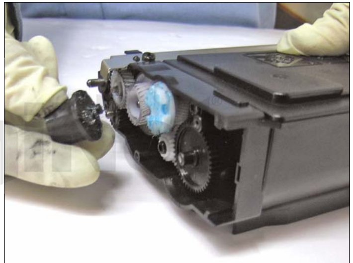
12. Extraer el engranaje externo (negro) como se muestra.
