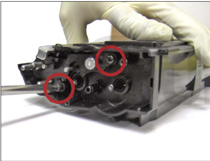
15. Aflojar los tres tornillos que sostienen la tapa lateral de los engranajes.
