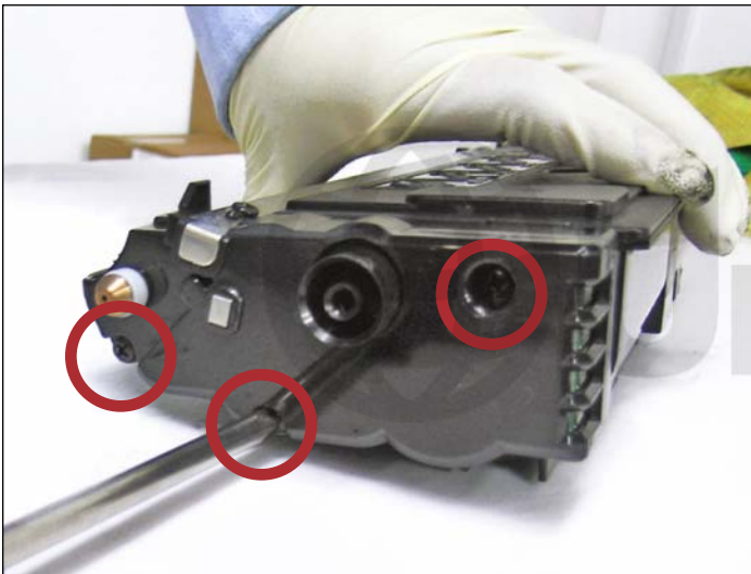
9. Aflojar los tres tornillos que sostienen la tapa lateral, lado sin engranajes.
