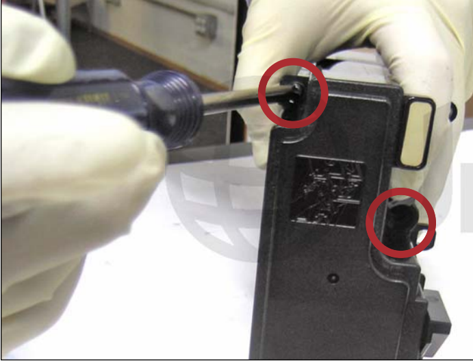
1. Retirar los dos tornillos que unen el depósito de desperdicios con el resto del cartucho.
