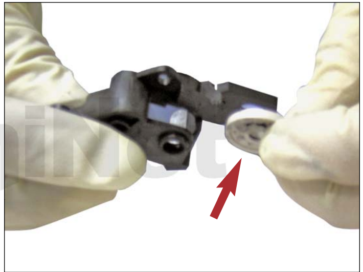
8. Juntar el buje blanco (derecha) con el soporte.
